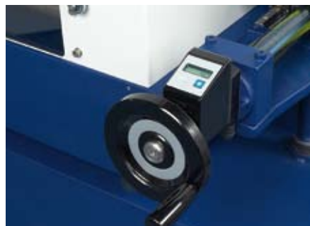
La manivelle de déplacement en X avec poignée de bridage (déplacement digital) facilite les coupes parallèles.
